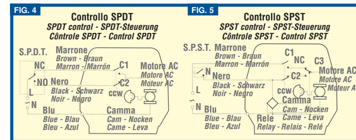
FIG. 4 Controllo SPDT SPDT control - SPDT-Steuerung Contrôle SPDT - Control SPDT
